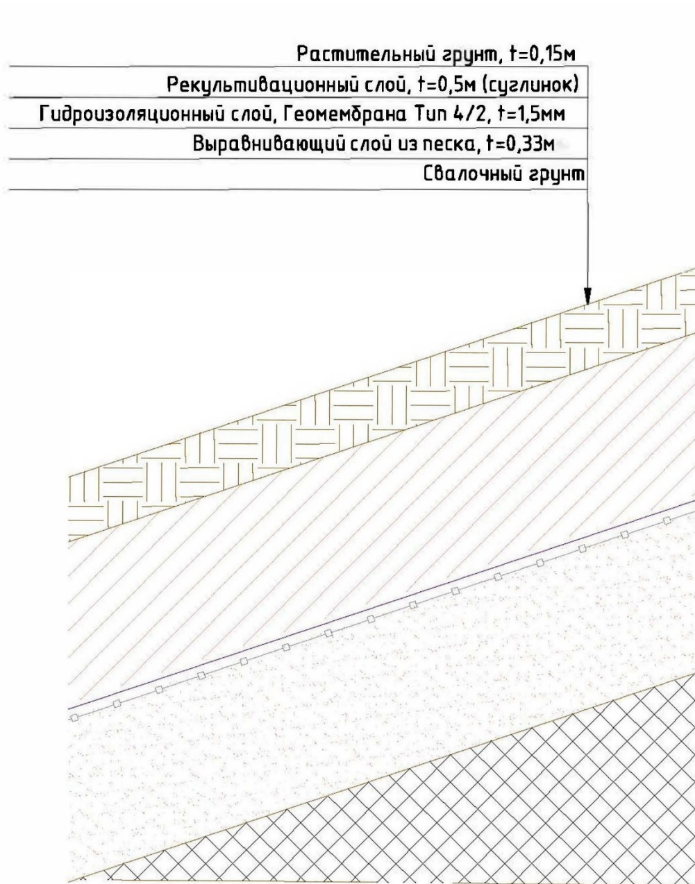
Рисунок 1 – Схема технической рекультивации несанкционированной свалки
