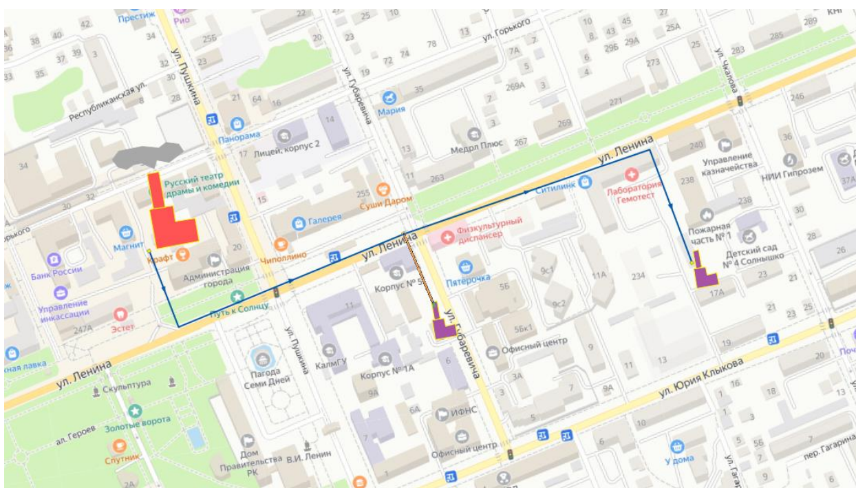
Рисунок 5.7.1 – Переключение нагрузки котельных «Юрия Клыкова» и «Совмин» на котельную «М. Горького» (зимняя, летняя)
