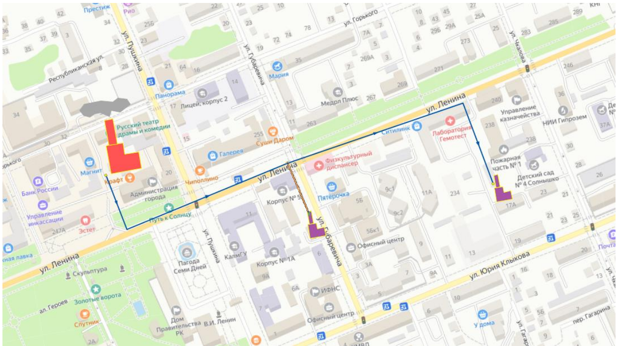
Рисунок 4.2.3 – Переключение нагрузки котельных «Юрия Клыкова» и «Совмин» на котельную «М. Горького» (зимняя, летняя)
