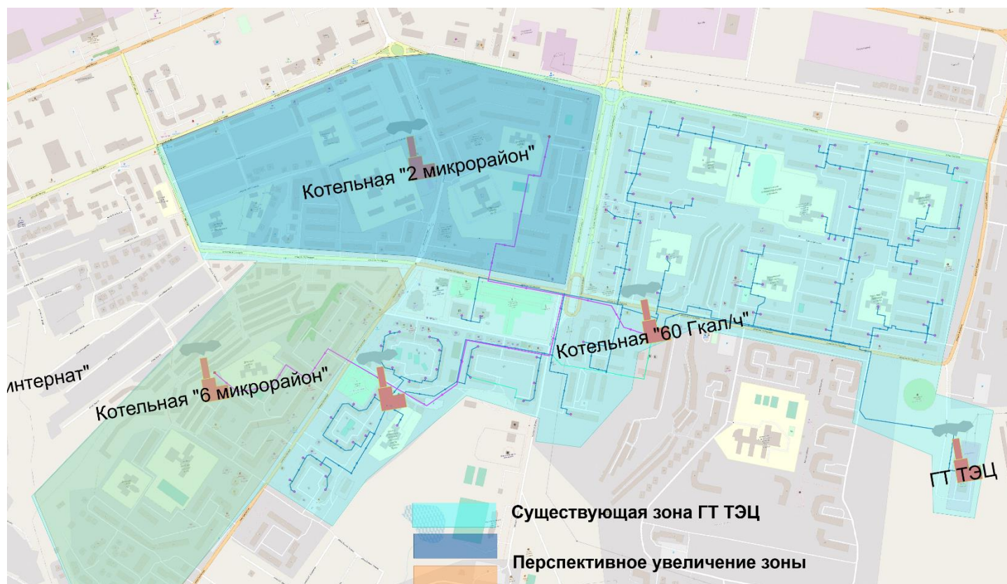
Рисунок 6.4.1 – Увеличение зоны действия Элистинской ГТ ТЭЦ при переключении на нее тепловой нагрузки двух котельных АО «Энергосервис» (Сценарий 1,2)
