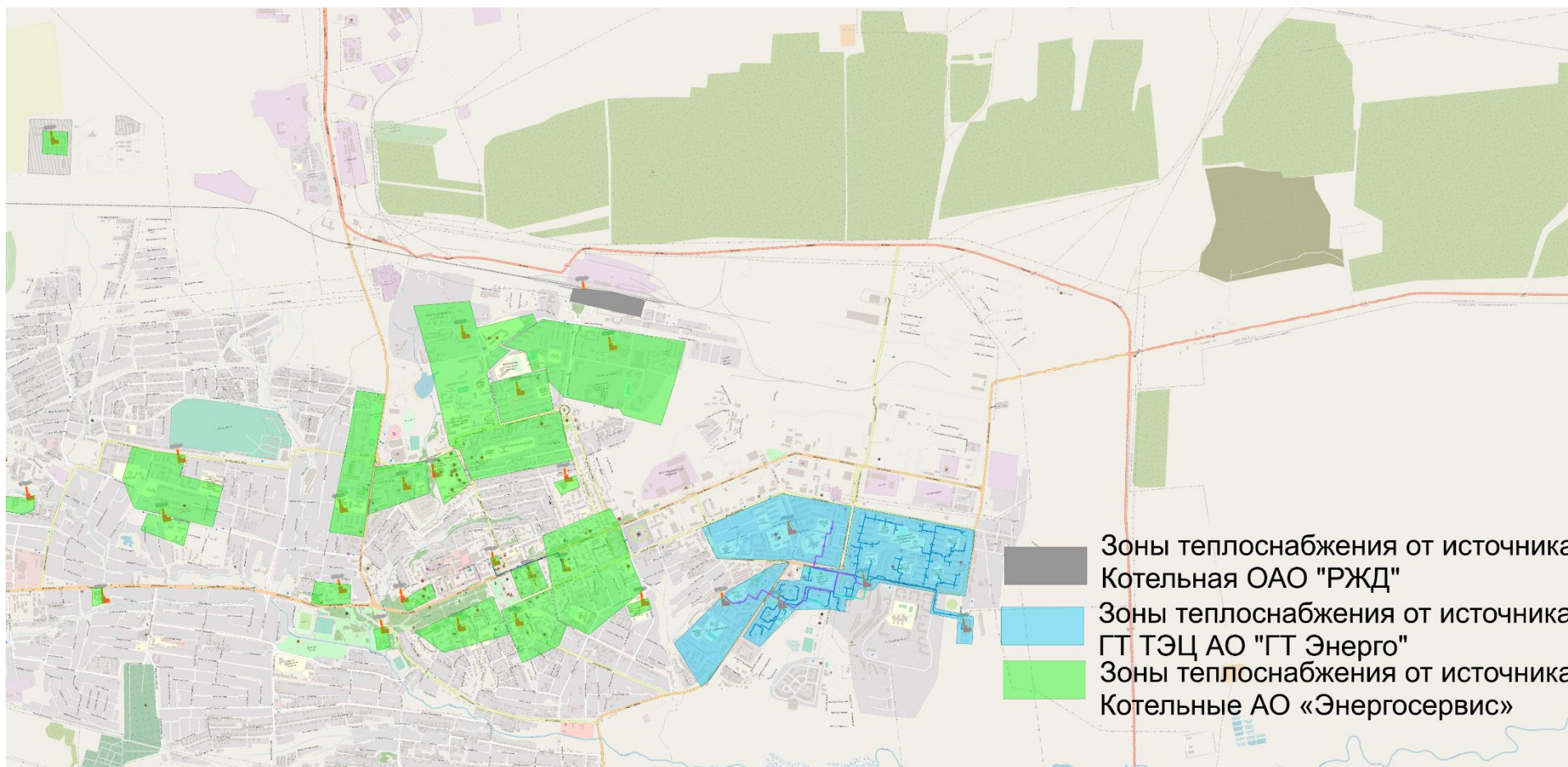
Рисунок 4.2.1 – Увеличение зоны действия Элистинской ГТ ТЭЦ при переключении на нее тепловой нагрузки двух котельных АО «Энергосервис» (Сценарий 1)
