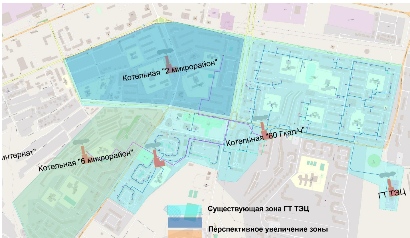
Рисунок 5.9.1 – Увеличение зоны действия Элистинской ГТ ТЭЦ при переключении на нее тепловой нагрузки двух котельных АО «Энергосервис» (Сценарий 1,2)
